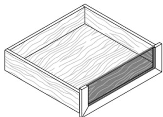
Height : 5 3/4"
